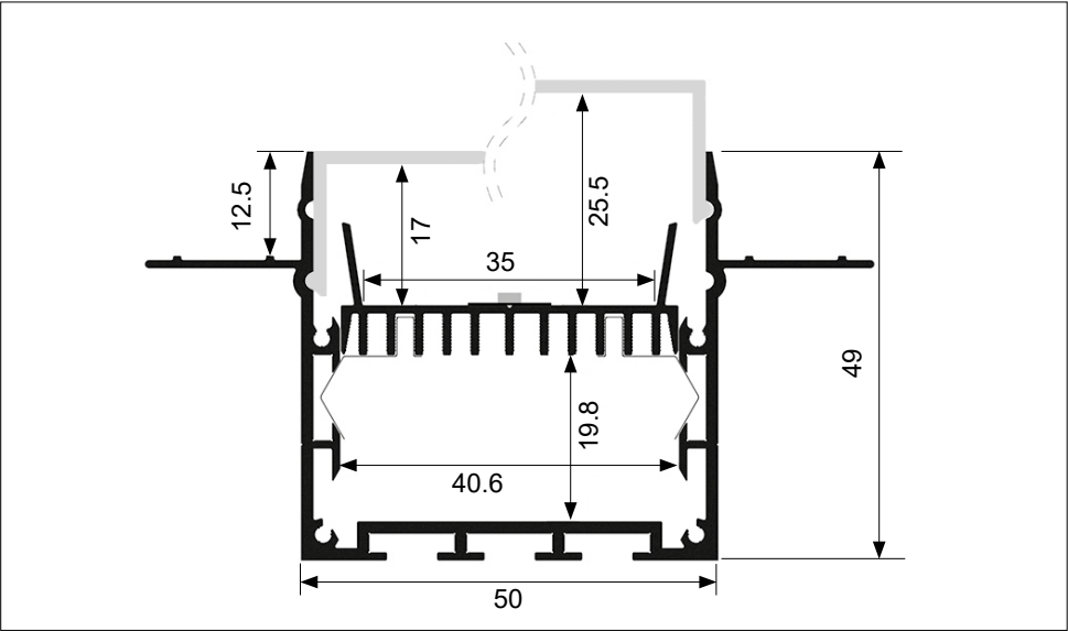
Difusor / Diffuser / Diffuseurs / Diffusore
