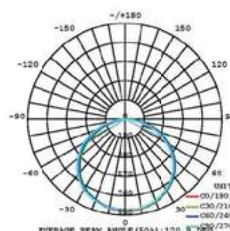
Curva Fotométrica Photometric curve
